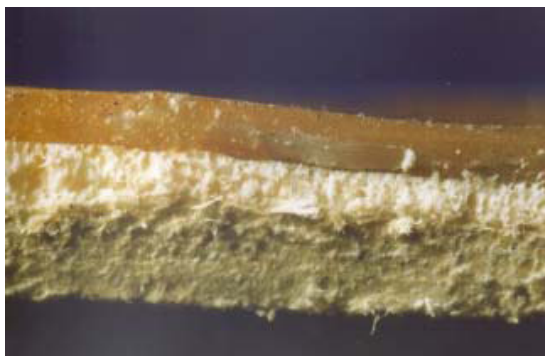
Coupe transversale d'un revêtement de sol posé dans les trains; couche inférieure en carton d'amiante
